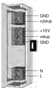
připojení – svorky
