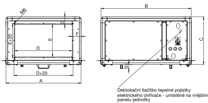
RME 2400; 3000; 4000; 6000 - poloha H1
