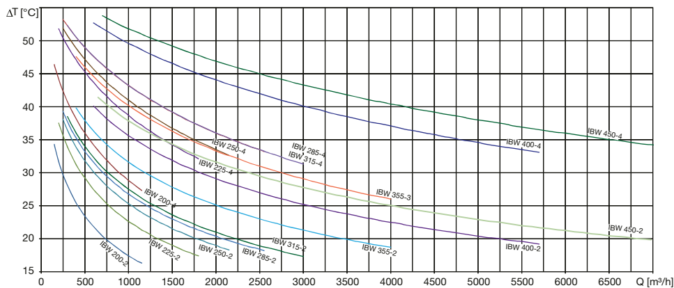
IBW – teplovodní ohřívače dT_w = 60/40^\circ\text{C}
