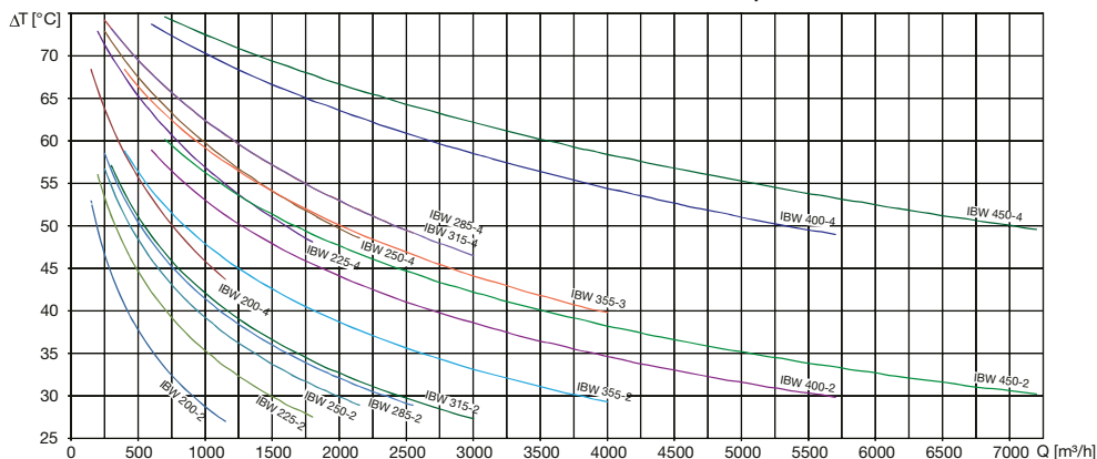
IBW – teplovodní ohřívače dT_w = 80/60^\circ\text{C}
