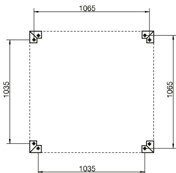
CAA 1100 (Ø1100)
