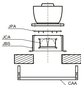
jednoduchý príklad montáže nasávanie strešného ventilátora
