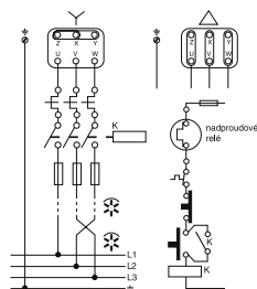
zapojení Y nebo \Delta podle typu a štítku na motoru
