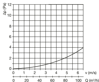
ED Flex® 90/75 EASY pre 1m rovného potrubia
