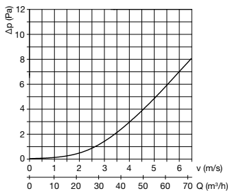
ED Flex® 75/63 PRO pre 1m rovného potrubia
