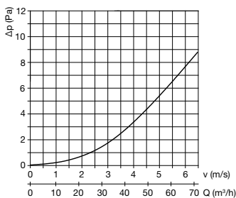
ED Flex® 75/63 EASY pro 1m rovného potrubia
