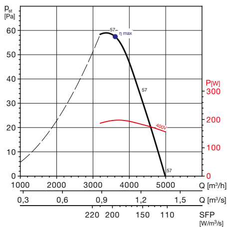
TCBT/6-500 H
