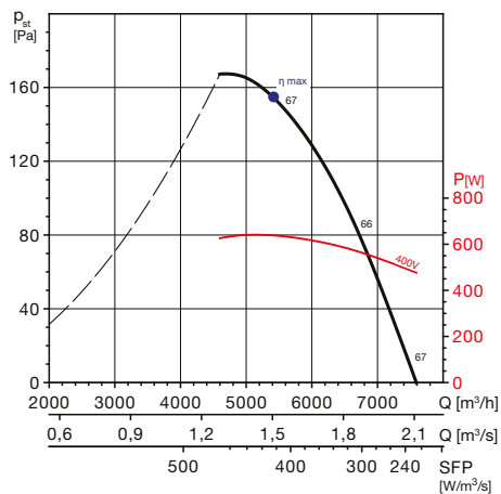
TCBT/4-500 H
