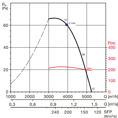
TCBB/6-500 H
