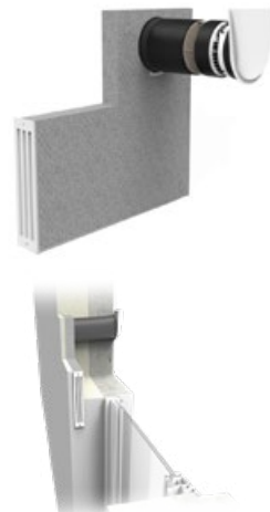
PULSE 160-W – skrytá inštalácia fasádnej mriežky v okennom ostení
