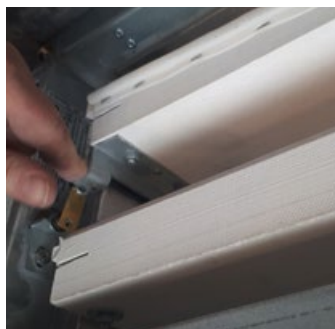
obrázek č. 11 – detail tepelné tavné pojistky u žaluziové klapy a jednotlivé polohy listu při aktivaci
