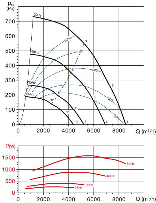
CRVT/4-500 N
