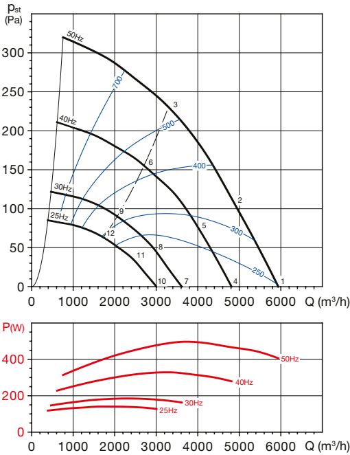
CRVT/6-500 N
