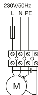
schéma elektrického zapojení
