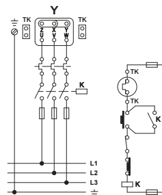
pripojenie ventilátora k sieti 3x400V
