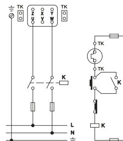
pripojenie ventilátora k sieti 1x230V
