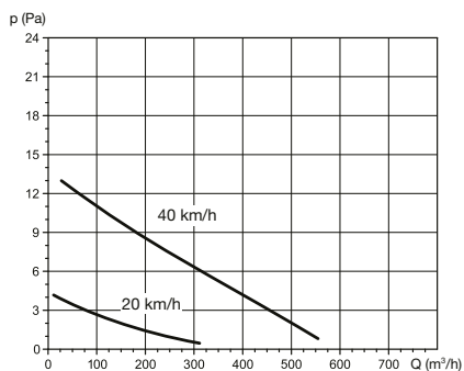
Tlakové charakteristiky strešnej hlavice VH 315 v závislosti od rýchlosti vetra (orientačné hodnoty)
