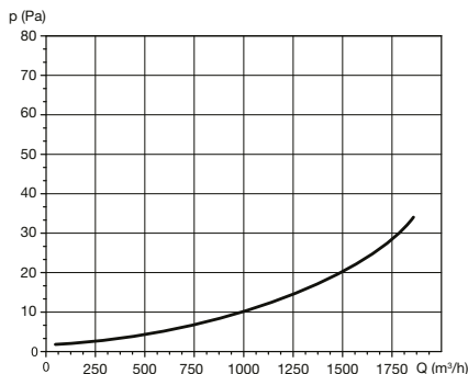
Hodnoty tlakových strát strešnej hlavice VH 315 v závislosti na prietoku vzduchu vo výtlačnom potrubí (orientačné hodnoty)
