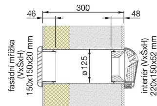
instalace přívodního prvku do stěny
