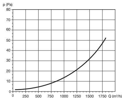
Hodnoty tlakových strát strešnej hlavice VHO 315 v závislosti od prietoku vzduchu vo výtllačnom potrubí (orientačné hodnoty)
