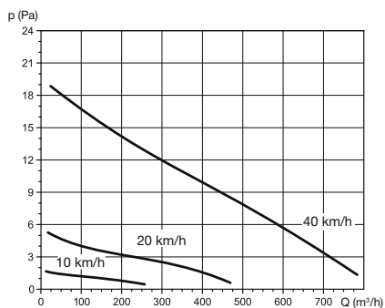
Tlakové charakteristiky strešnej hlavice VHO 315 v závislosti od rýchlosti vetra (orientačné hodnoty)
